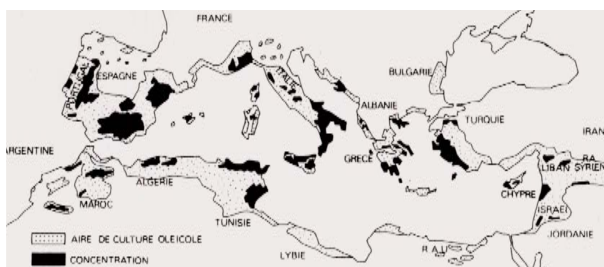
Figure 2 : Les principaux pays oléicoles du bassin méditerranéen [9]
