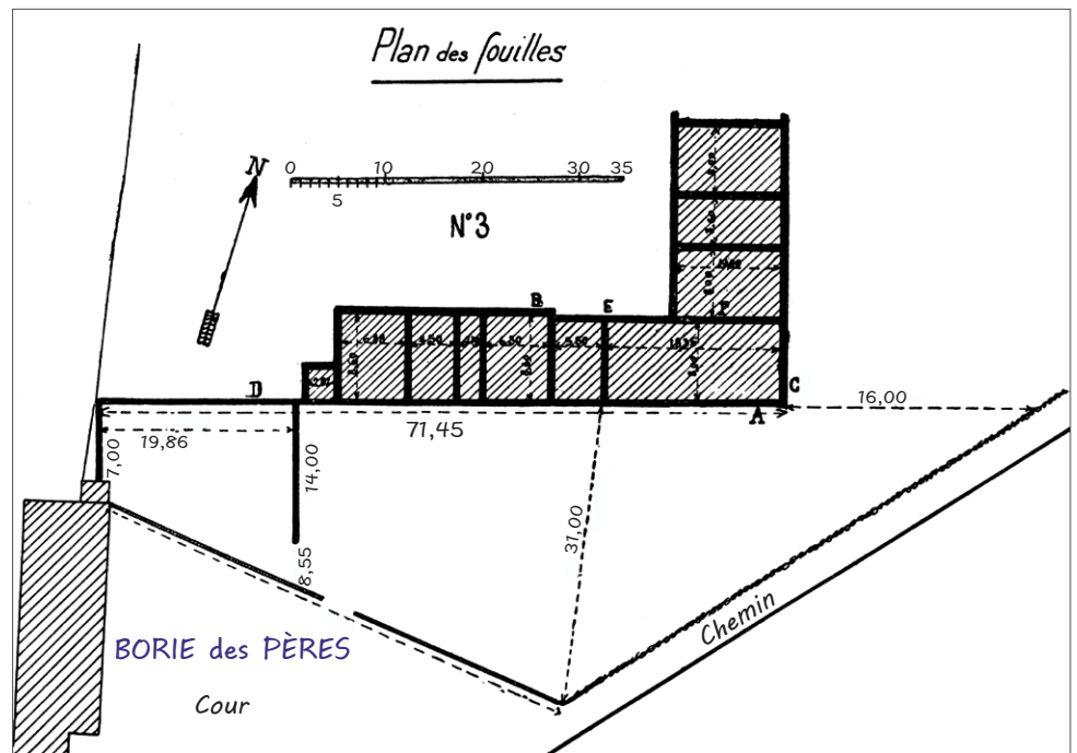
6 - Plan de La Borie des Pères à Villefranche-de-Rouergue d'après P. BORIES
