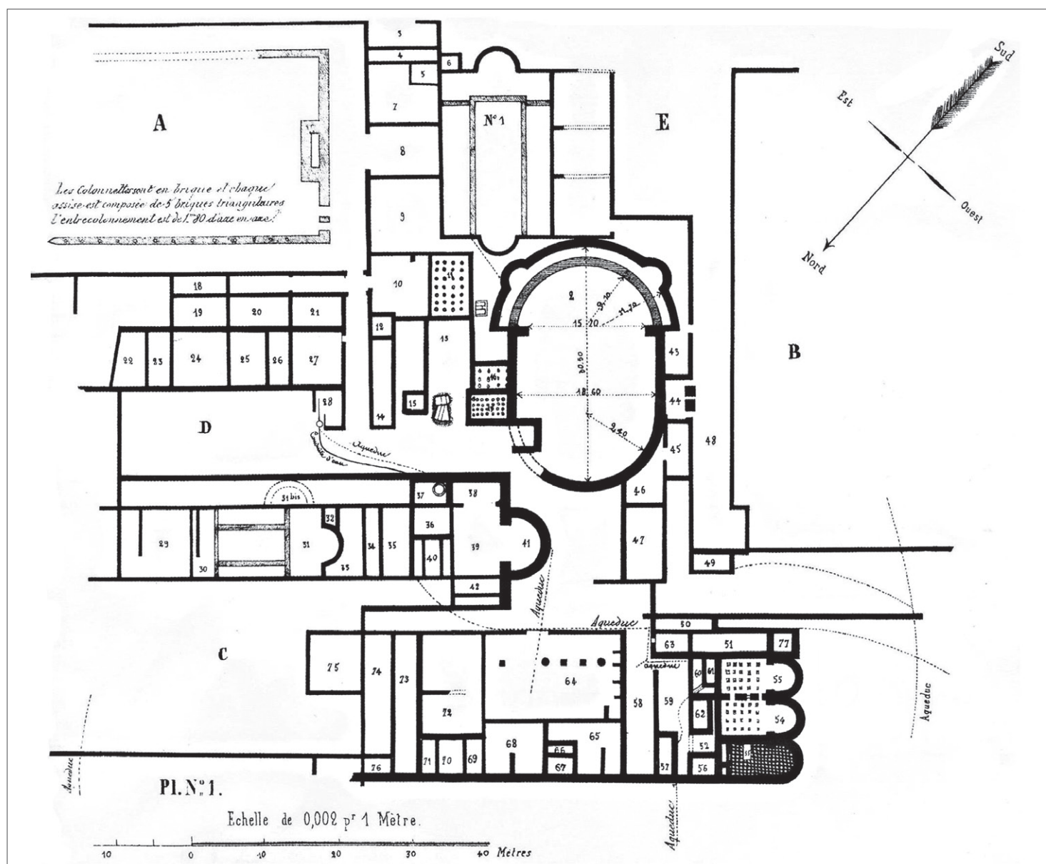
5- Plan de la villa Argentea à Montrozier selon l'Abbé CÉRÈS.
