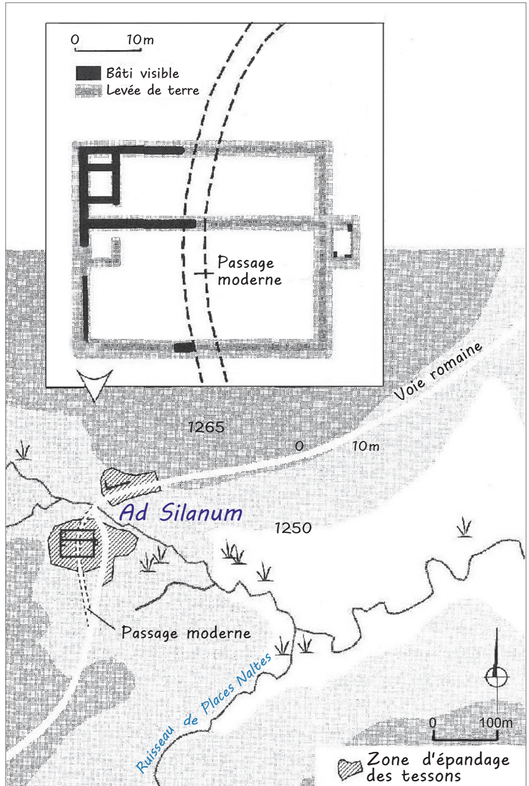
10 - Plan des vestiges de la Station d'Ad Silanum (DIEULEFAIT 2006)
