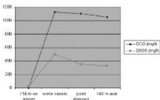
Figure n°7 : variation de la DCO et DBO5 dans la rivière Mfoulou.
