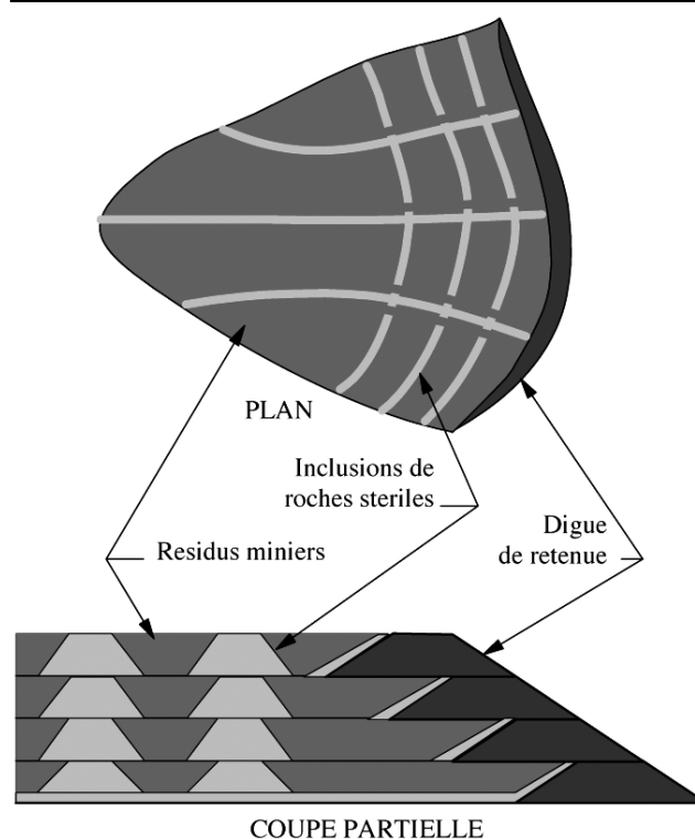
Figure 1. Inclusions de roches stériles placées dans un parc à résidus miniers (basé sur le concept proposé par Aubertin et al., 2002b, et développé par James et Aubertin, 2010, 2012).
