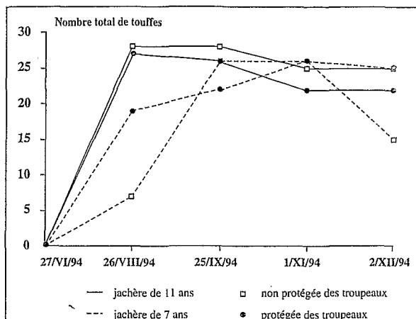
FIG 4.- Evolution de l'effectif des touffes de Andropogon gayanus entre deux et cinq mois après le semis de 1000 graines dans deux parcelles désherbées de jachère (Bondoukuy, Burkina Faso).
