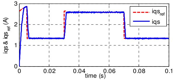
Fig. 7. Optimal currents i_{ds}, i_{qs}
