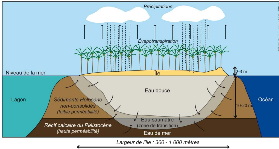
Figure 4 : Coupe transversale, verticalement exagérée, schématisant la structure de la lentille d'eau douce d'une île récifale.
