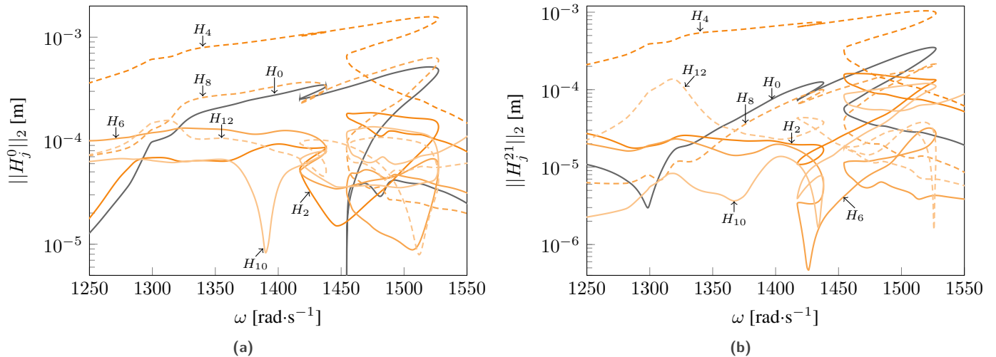
Figure 20 – Harmonics contribution for RL-HBM radial displacements solutions at (a) LE and (b) TE: H_0 (—), H_2 (—), H_4 (---), H_6 (—), H_8 (---), H_{10} (—) and H_{12} (---).
