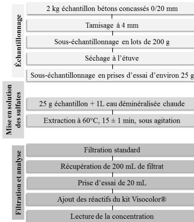
Figure 2 : Étapes de détermination des sulfates solubles dans les matériaux de construction
