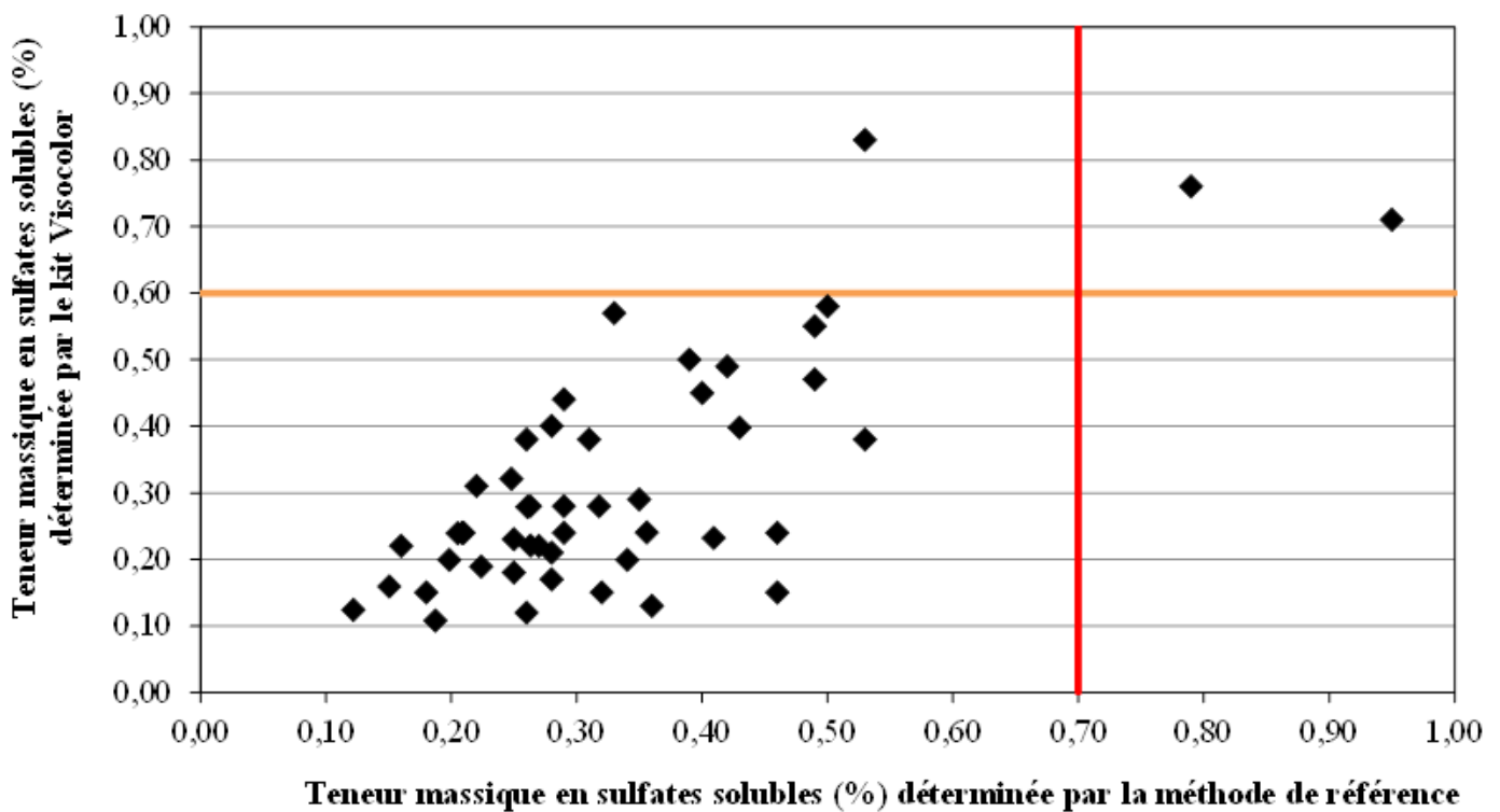
Figure 3 : Corrélation des teneurs en sulfates solubles obtenues par la méthode de référence et par le kit Visocolor® dans des échantillons de bétons concassés
