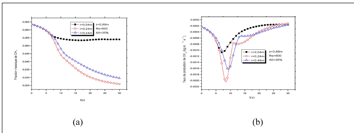
Figure 8. Evolution au cours du temps de la fraction massique (a) et du taux de production (b) de CH 4 en régime laminaire
