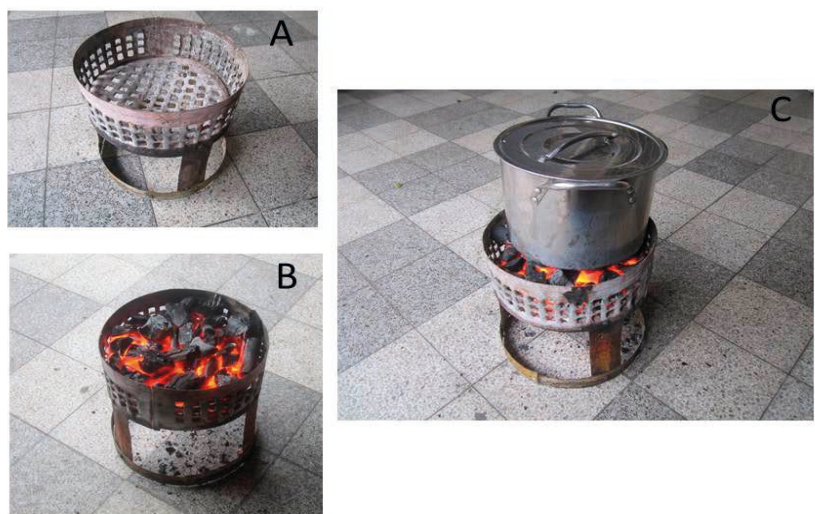
Figure 2. Foyer de cuisson amélioré ICS 16/8/C.
