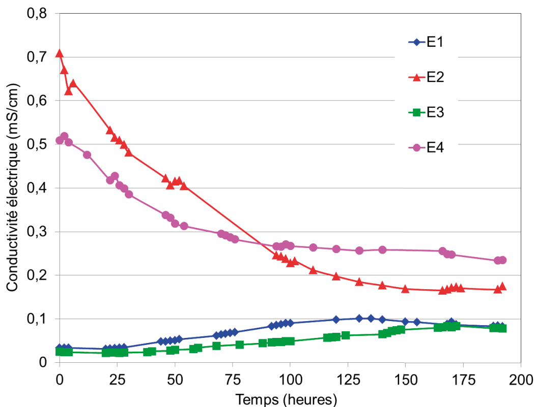
Figure 2. Évolution de la conductivité électrique des matériaux étudiés en fonction du temps.
