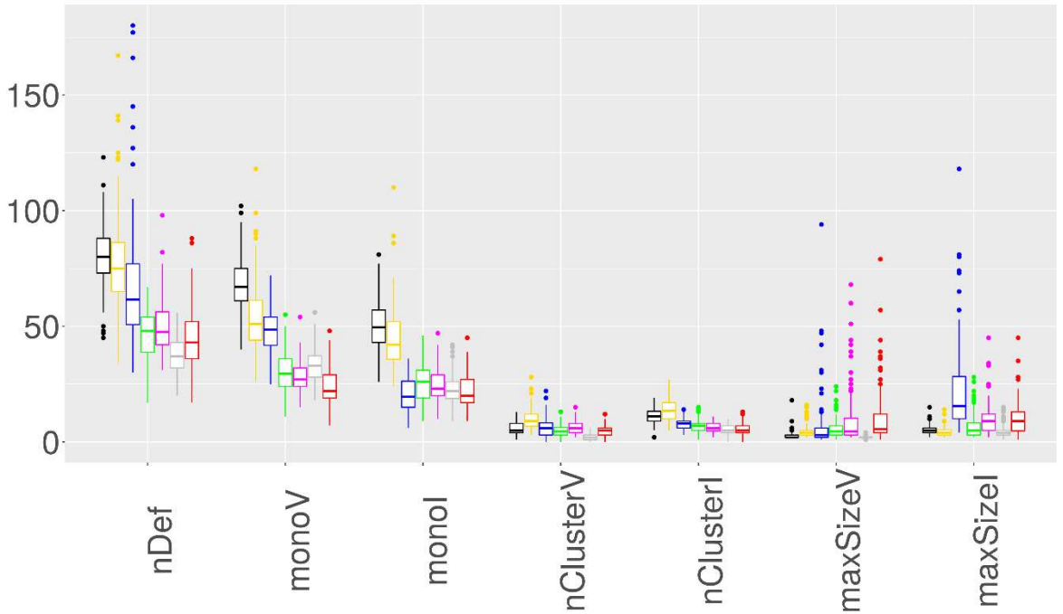
(b) W
