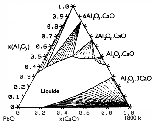
Figure 5 : Coupe isotherme du système Al 2 O 3 -CaO-PbO obtenue à la température de 1800 K. (les compositions sont exprimées en fractions molaires et les températures en Kelvins)
