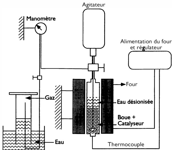
Figure 1 : Schéma expérimental
