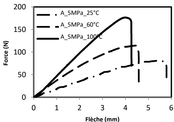
Figure 9. Courbe type force-flèche de CBPo en flexion à différentes température (échantillons compactés à 5MPa)
