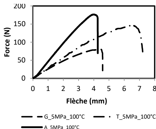
Figure 10. Courbe type force-flèche de CBPo en flexion pour différentes espèces séchées à 100°C (G : Gmelina ; A : Afzelia ; T : Teck ; (échantillons compactés à 5MPa).
