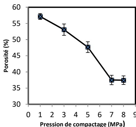
Figure 7. Evolution de la porosité des CBPo en fonction de la pression de compactage, (échantillons à base de sciure de Gmelina séchés à 25 °C).
