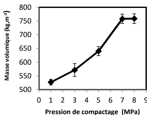
Figure 6. Evolution des caractéristiques mécaniques du CBPo en fonction de la pression de compactage, (échantillons à base de sciure de Gmelina séchés à 25°C).
