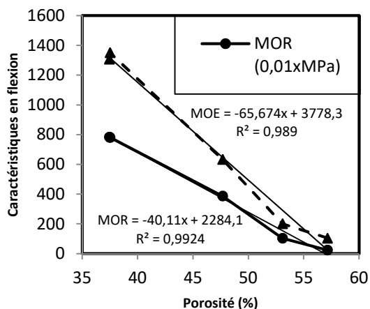
Figure 8. Evolution du MOE et du MOR des CBPo en fonction de la pression de compactage, (échantillons à base de sciure de Gmelina séchés à 25 °C).
