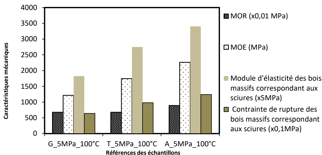
Figure 13. Valeurs comparées de MOE et MOR des CBPo à base de sciures de différentes espèces de bois, avec les modules et contraintes des bois massifs correspondants (G : Gmelina ; T : Teck ; A : Afzelia )
