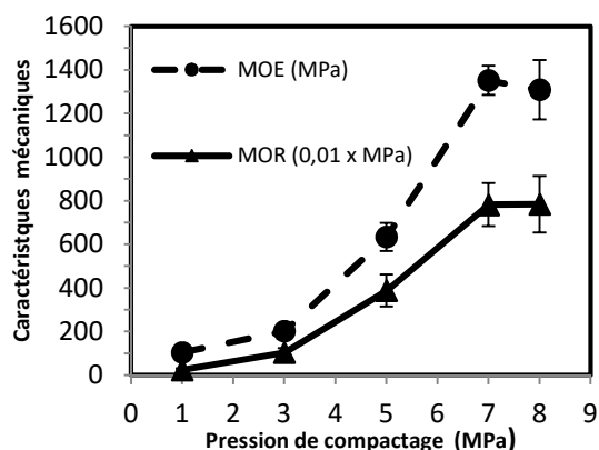
Figure 5. Evolution des caractéristiques mécaniques du CBPo en fonction de la pression de compactage, (échantillons à base de sciure de Gmelina séchés à 25°C).
