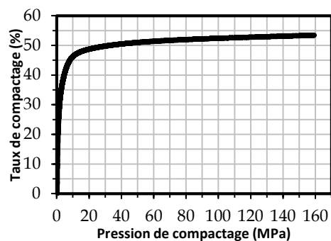
Figure 3. Evolution du taux de compactage en fonction de la pression.
