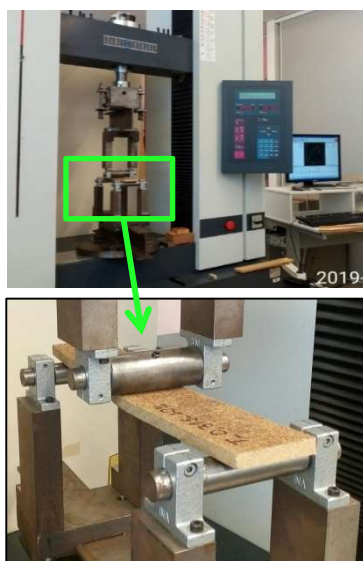
Figure 2. Dispositif expérimental pour l'essai de flexion
