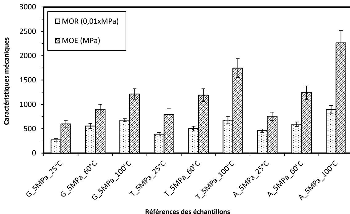
Figure 11. Valeurs comparées de MOE et MOR des CBPo, pour les 3 températures et les 3 espèces de bois (échantillons compactés à 5 MPa).
