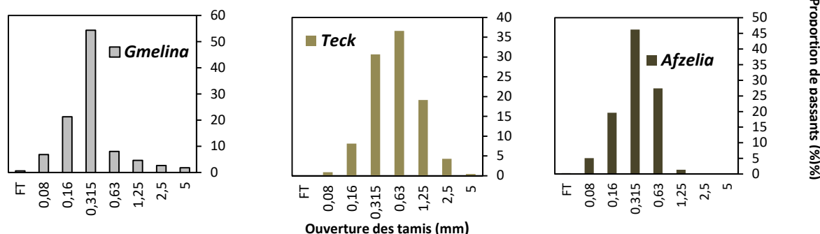
Figure 1. Distribution granulométrique des sciures de Gmelina , Teck et Afzelia .
