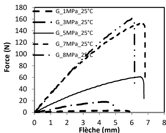
Figure 4. Courbe force-flèche du CBPo en flexion, pour différentes valeurs de pression de compactage, (échantillons à base de sciure de Gmelina séchés à 25 °C)
