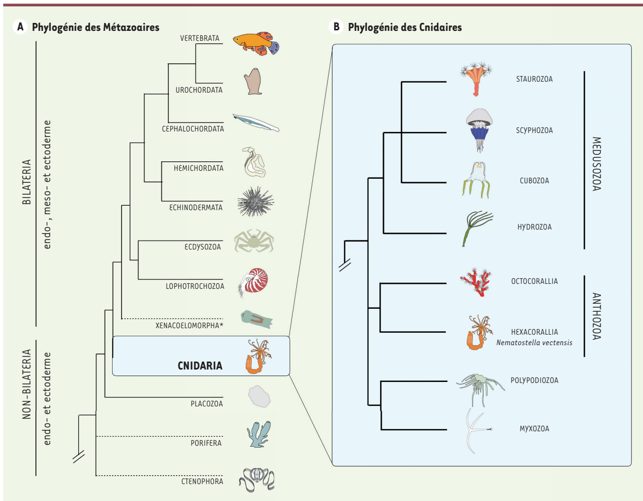
Figure 1. Phylogénie simplifiée des métazoaires (animaux). A. Phylogénie des métazoaires, mettant en évidence la position clé des cnidaires en tant que groupe frère des animaux bilatériens. La position des cténophores et porifères à l’extérieur des bilatériens reste controversée (lignes en pointillés). B. Phylogénie des cnidaires, illustrant les relations entre les principaux groupes (figure modifiée à partir de [11]).
