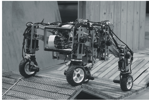
Fig. 1. HyLoS Robot
