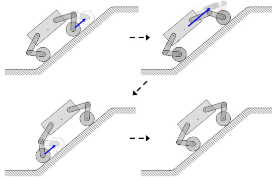
Fig. 3. Peristaltic mode
