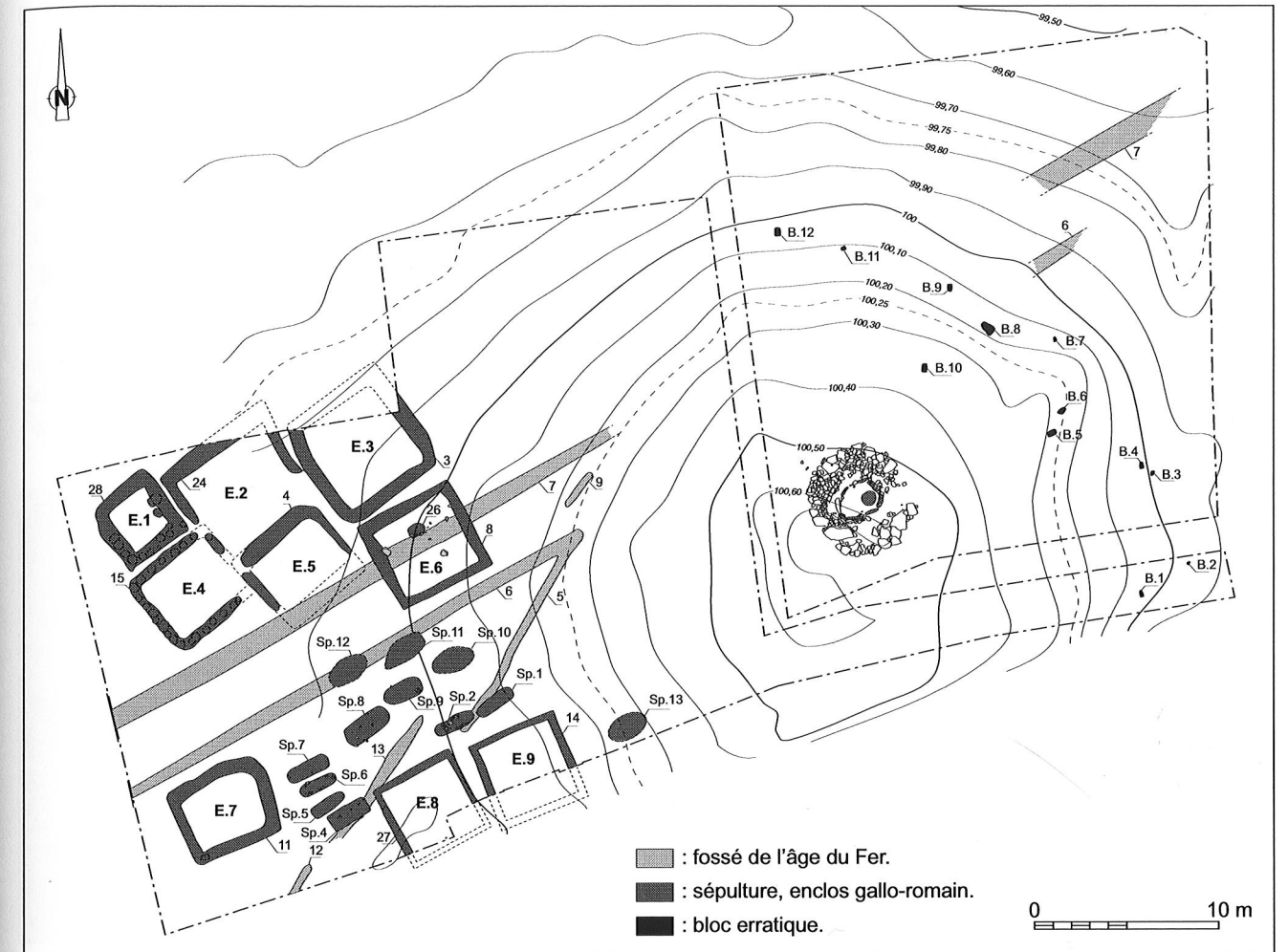
Figure 3 : Gouesnac'h Ty Korn. Plan général du site et microtopographie du terre funéraire (altitudes relatives en mètres). Infographie S. Jean.
