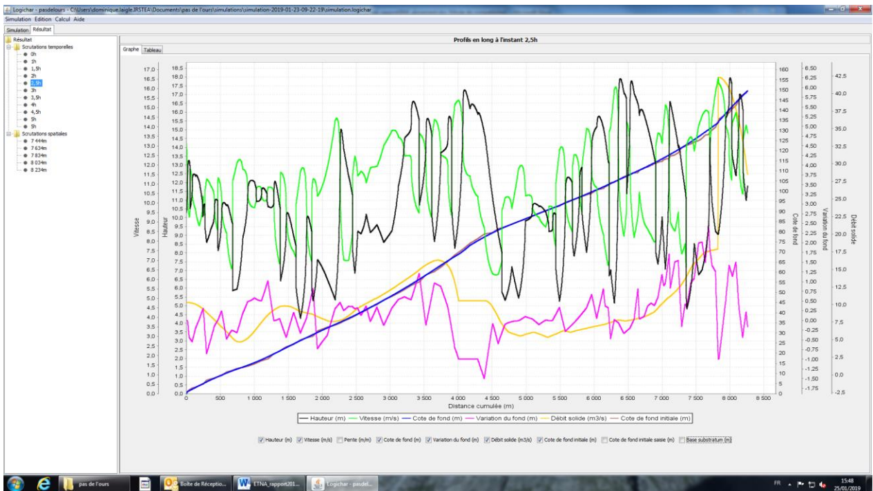
Figure 42 : Profils à 2,5 h de hauteur, vitesse, débit solide et évolution du fond par rapport à la situation initiale (hyd. Rub 3 – 40 m)
