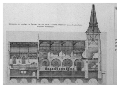
Fig. 2 : Howard Robertson, projet de diplôme : une église pour le culte anglican, coupe longitudinale, Bulletin hebdomadaire de la SADG , 1913, p. 346.
