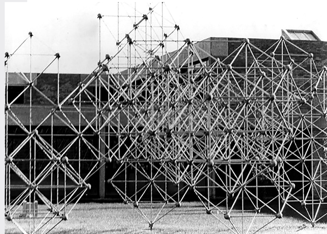
Fig. 4 : Sculpture en structure aluminium au Centre des conducteurs de travaux à Labège (P. Gardia et M. Zavagno arch.), réalisée par l'Atelier supérieur de sculpture de l'école des beaux-arts de Toulouse : A. Blanchard, J.-P. Bouglon, J.-J. Durancet et G. Tiné, 1968-1969. Ph. J.-P. Bouglon.
