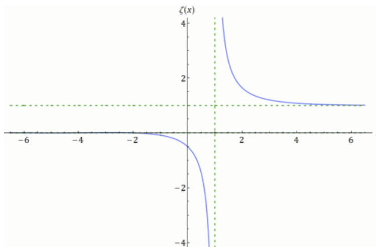
FIGURE 1 – Graphe de la fonction zêta
