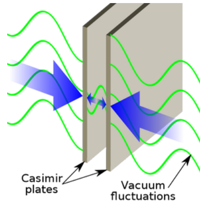
FIGURE 2 – L'effet Casimir
