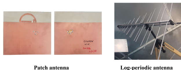
Fig. 1. Measurement antennas.
