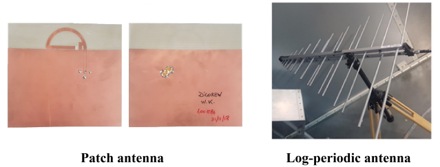
Fig. 1. Measurement antennas.
