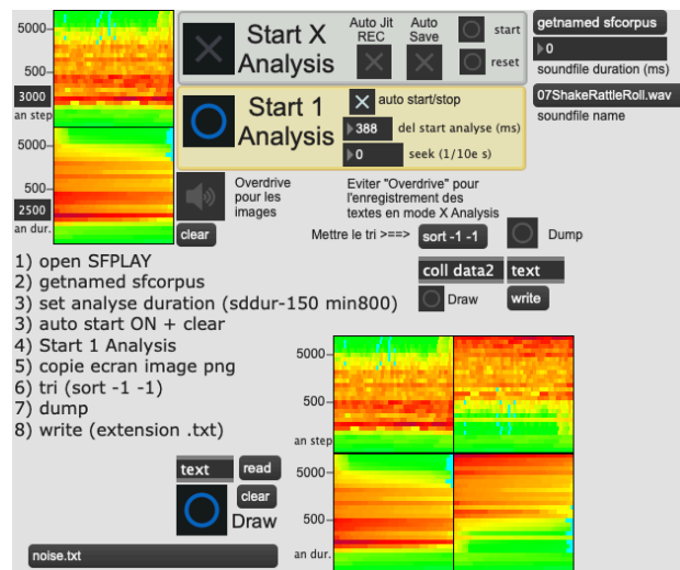
Figure 13. La visualisation successive des signatures en temps réel (pendant la lecture des sons), et les différentes modes : analyse simple ( I Analyses ), analyse d'un morceau entier ( X analysis ), d'un répertoire ( getnamed sfcopus ).
