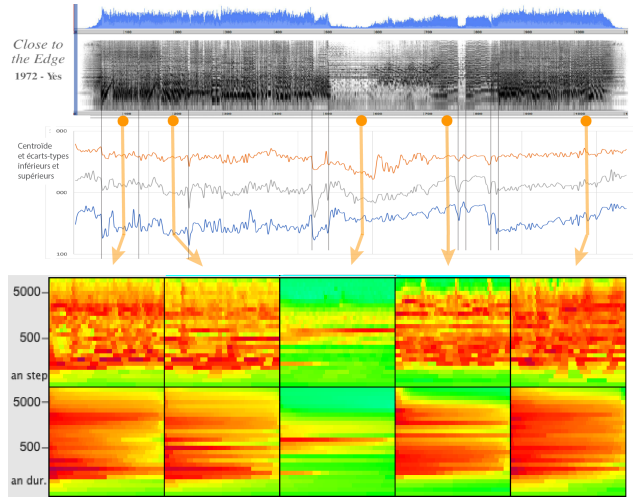
Figure 16. Close to the Edge , de haut en bas : enveloppe, spectrogramme, graphe du centroid et des écarts, signatures à quelques instants clés.
