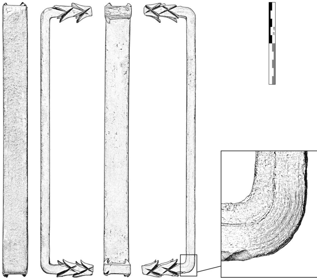
Figure 8 : Crampon formé par laminage.
