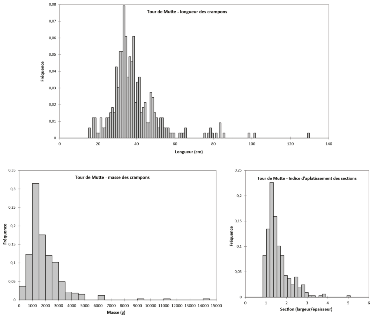
Figure 4 : Distributions des longueurs, masses et rapports d'aplatissement des crampons prélevés.
