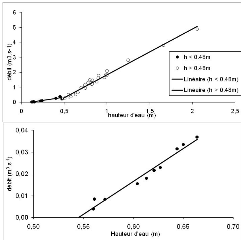
Figure 18 – Courbes de tarage établies pour la Goule (haut) et le Diabie (Bas) à partir de mesures ponctuelles de débits réalisées durant trois étés successifs (2008, 2009 et 2010).
