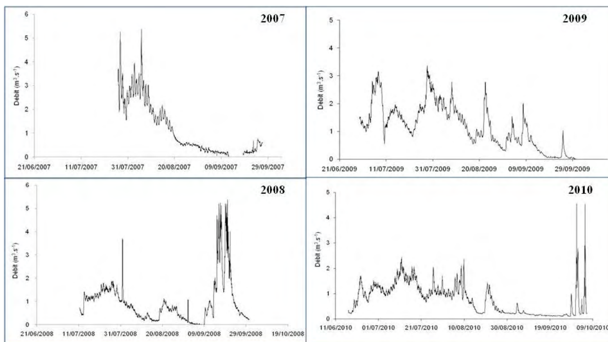
Figure 21 – Suivi du débit de la Goule durant les étés 2007, 2008, 2009 et 2010. Les hydrogrammes diffèrent fortement d'une année à l'autre car liés à la variabilité des paramètres climatiques : la température de l'air contrôle la fonte et la pluie contribue directement et rapidement aux écoulements, spécialement en fin de saison lorsque le sol est déjà gelé.
