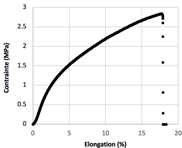
Fig. 2 : exemple d'une courbe de traction (film MFC/P35)
