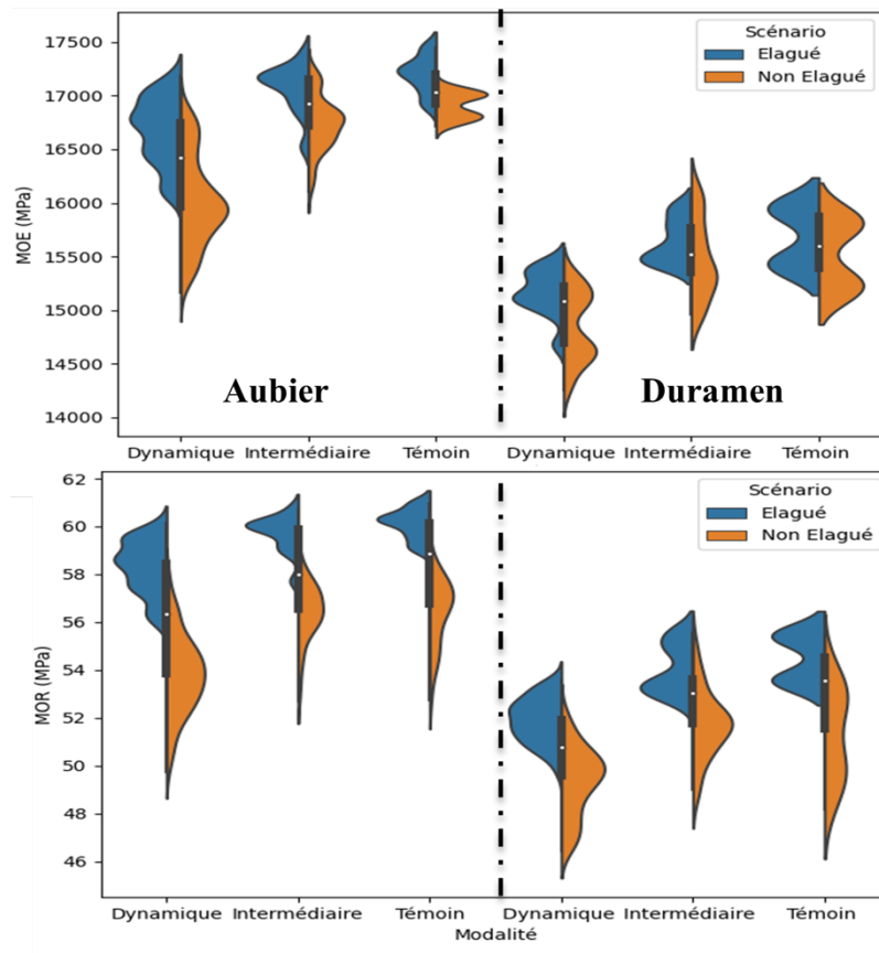
Fig. 5 : Comparaison des propriétés mécaniques entre les poutres LVL constituées d'arbres élagués et les poutres LVL constituées d'arbres non élagués
