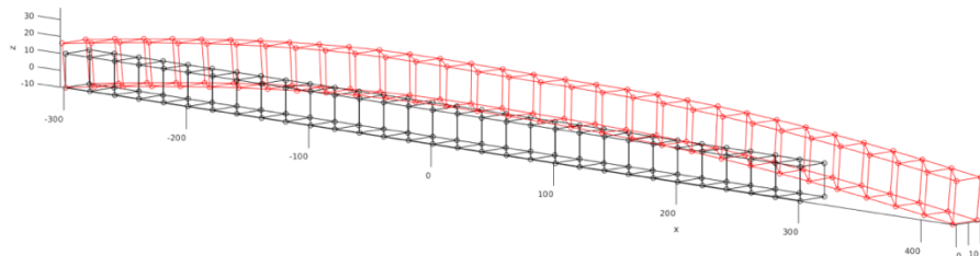
Fig. 4 : calcul de flèche sur dosse par un élément de solide-coque.
