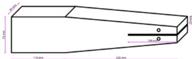
Fig.2 : Eprouvettes pour l'essai de fissuration
