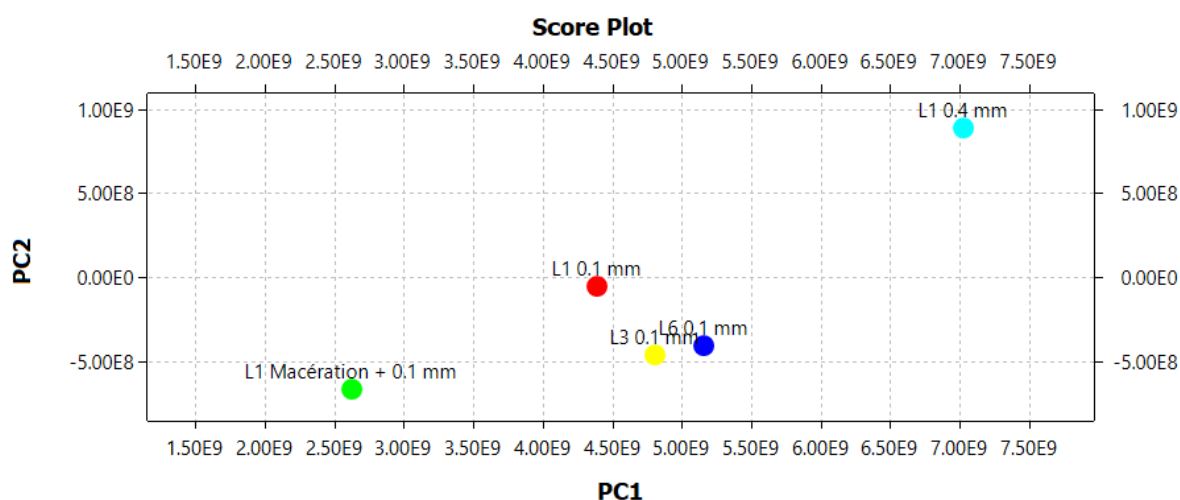
Fig. 1 : Analyse en composante principale de la granulométrie des pyrolysats et des minéraux sur les produits de dégradation du hêtre. Est représenté le résultat d'une PCA sur différents échantillons de l'écorce d'un seul hêtre. PC1 explique 85% de la variance et PC2 en explique 13%. Les échantillons sont décrits selon 3 critères : la hauteur de l'arbre, la granulométrie et la macération. L indique différentes hauteurs (L1 = 0,3 m ; L3 = 1,3m ; L6 = 14,85m)
