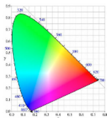
Fig. 2 : Diagramme de chromaticité
