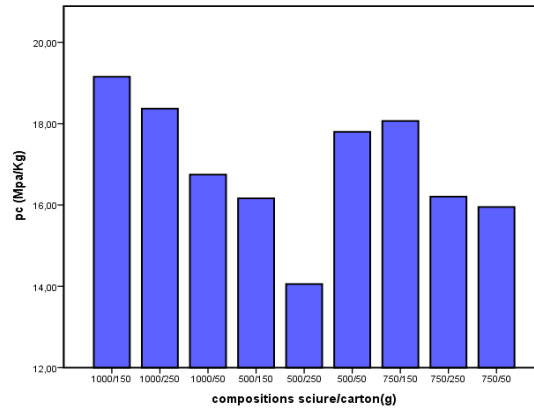
Fig. 5 : Pouvoir calorifique des échantillons
