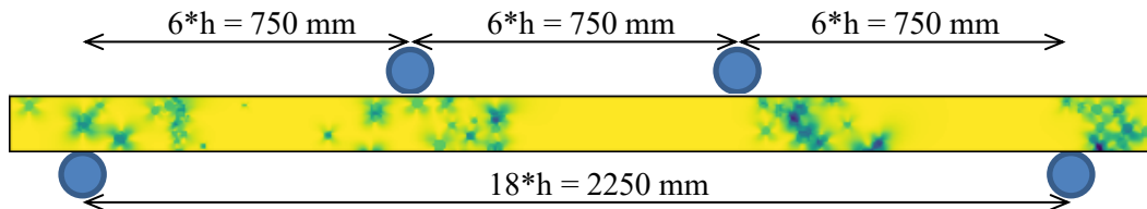
Fig. 4 : Spécification de l'essai de flexion virtuel suivant la norme EN 408
