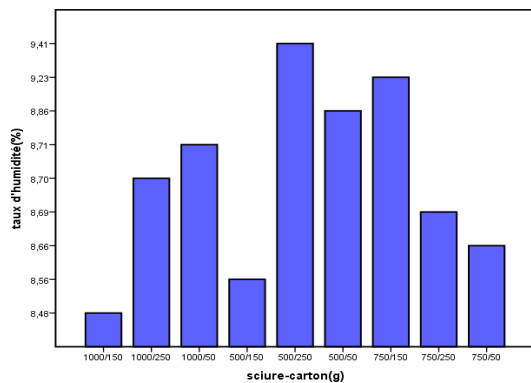
Fig. 3 : Humidité des échantillons
