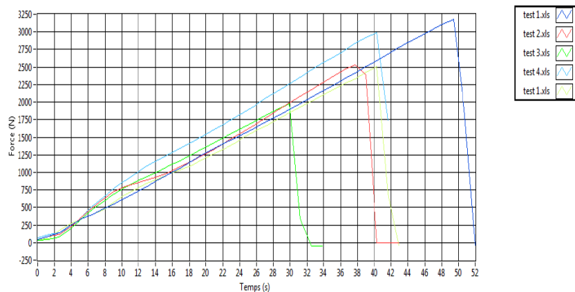
Fig.3 : Test de traction des panneaux de contreplaqués collés avec des colles biosourcées.
