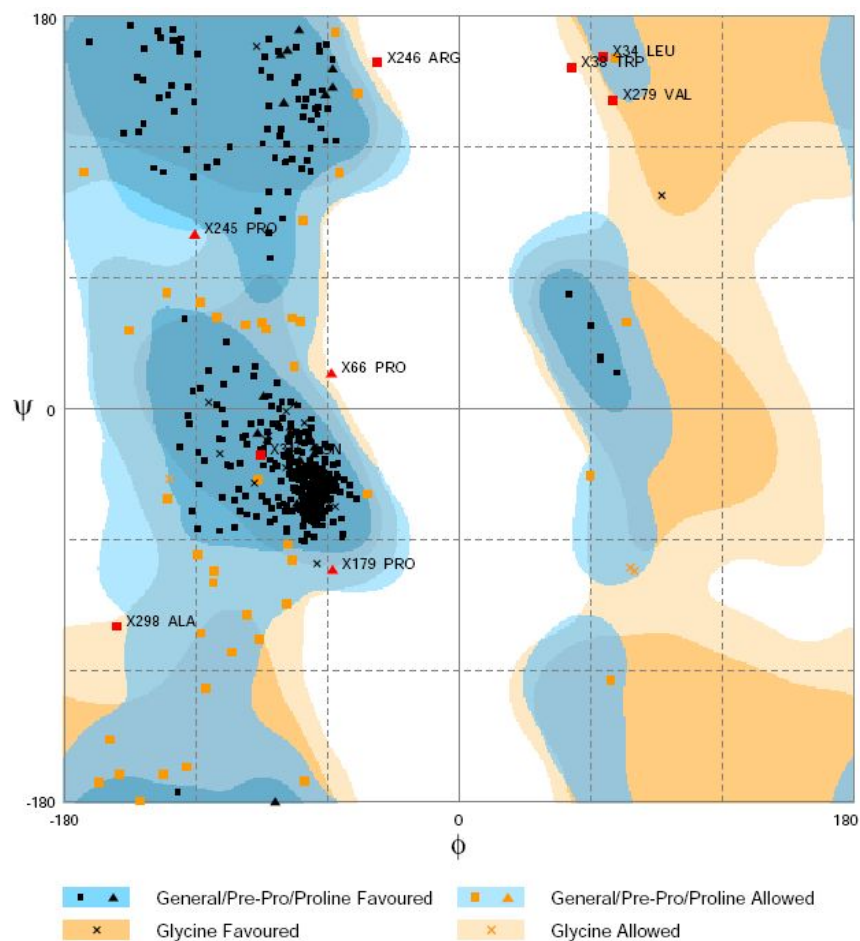
Figure 6. Ramachandran plot of the « RFVT3-3WDO » model
