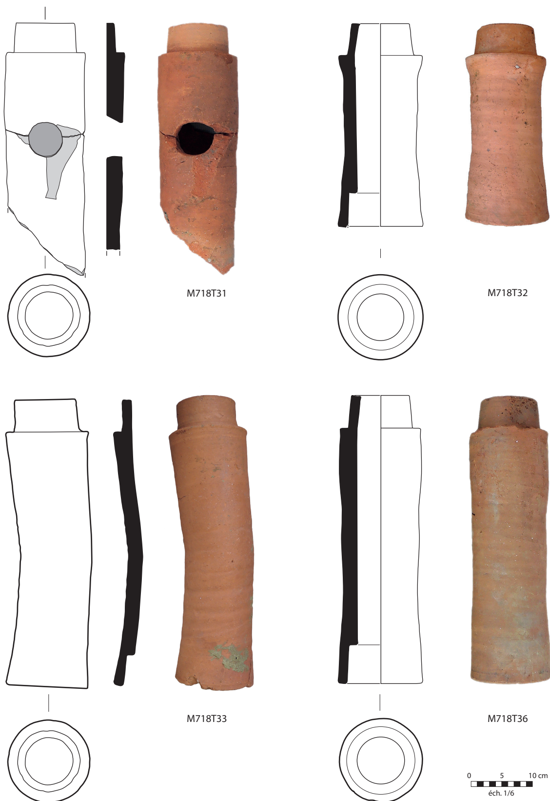
Fig. 7. Relevés de quatre cylindres issus de la conduite en terre cuite CN 660 : cylindre à l'orifice, cylindre court, cylindre coudé et cylindre standard (C. Chaze et J. Ramona, SAVL).
