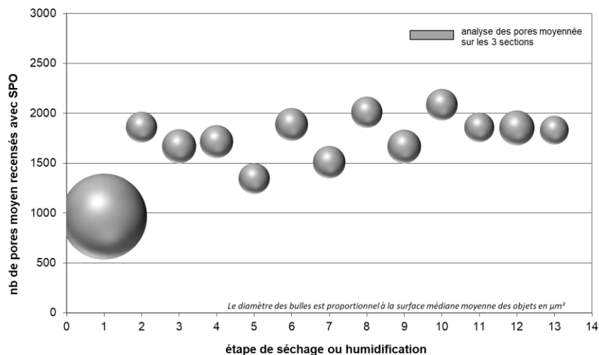
Figure 6. Évolution du nombre et de la taille des pores à chaque étape de séchage et d'humidification sur la moyenne des 3 sections étudiées.
