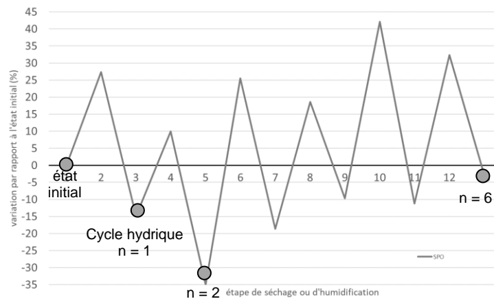
Figure 5. Évolution de la porosité moyenne de l'échantillon à chaque étape de séchage et d'humidification (avec n = nombre de cycles hydriques complets) avec le logiciel SPO.
