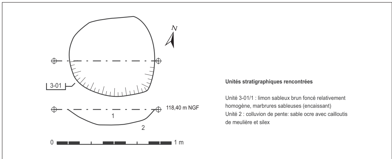
Fig. 41 Relevé en plan et coupe de la fosse 3-01.
