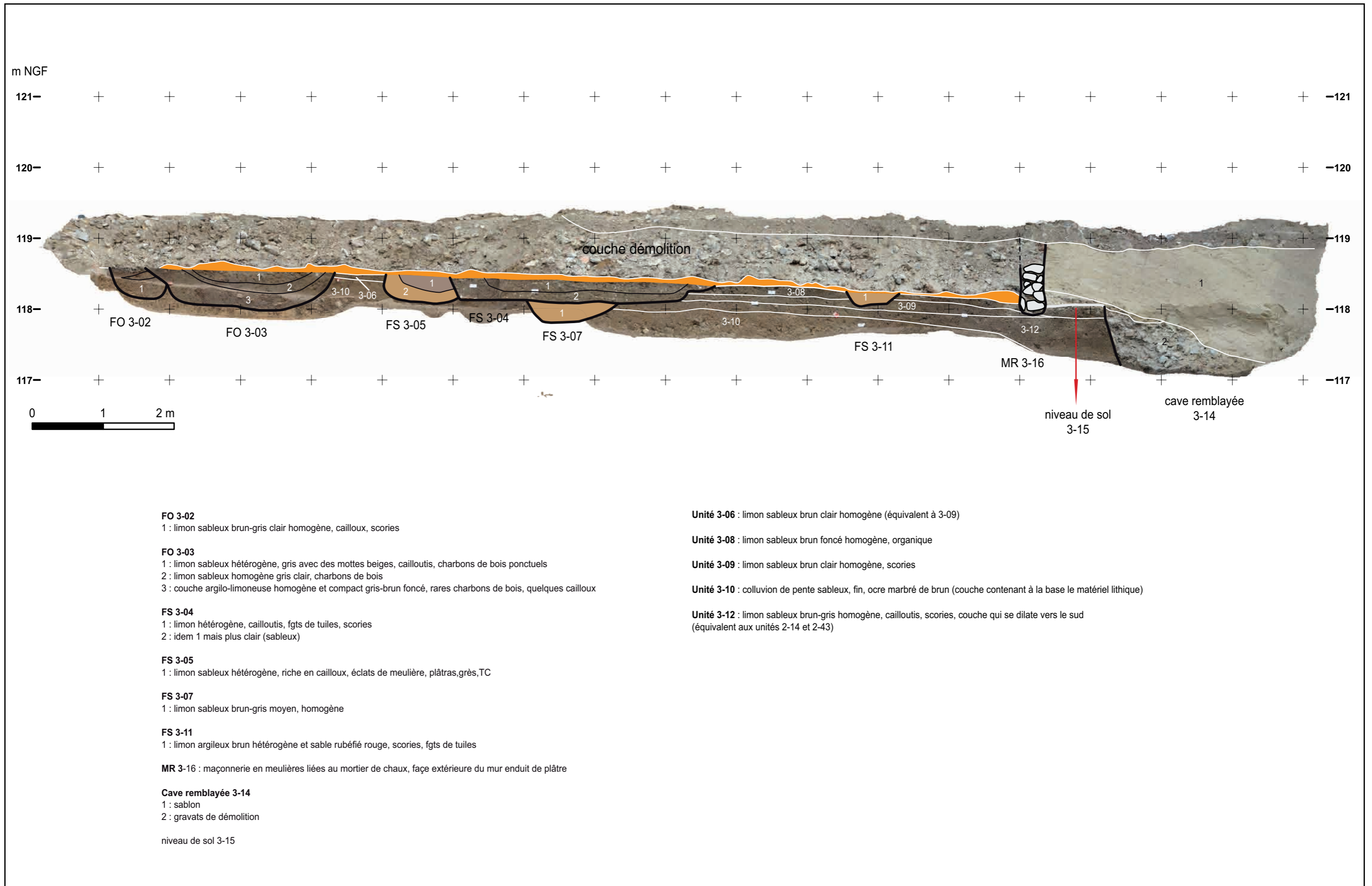
Fig. 35 Coupe photogrammétrique de la bordure orientale de la tranchée 3. Traitement photogrammétrique : M. Belarbi, Inrap ; DAO : N. Warmé, Inrap
