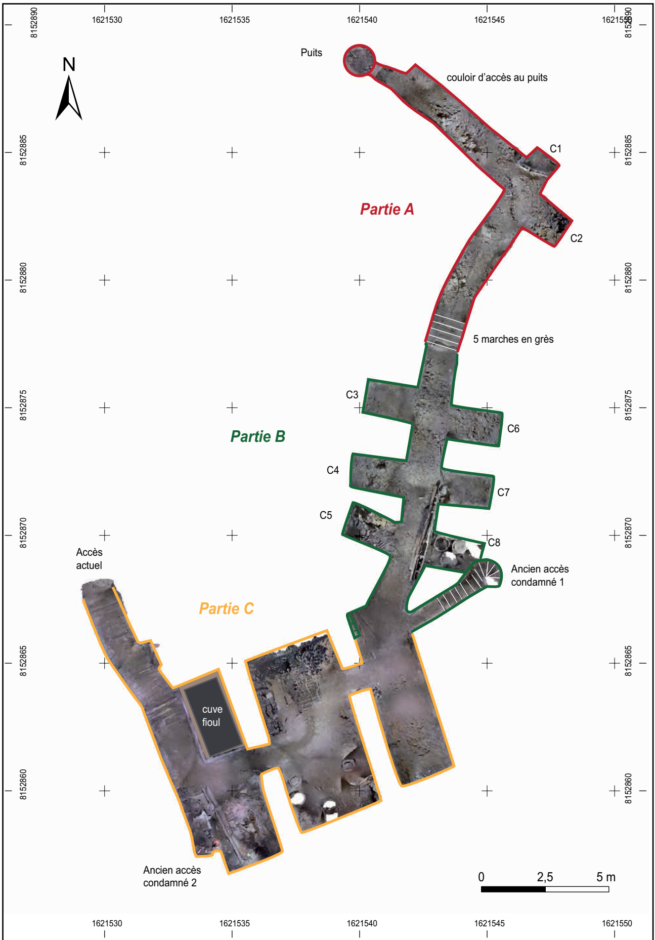
Fig. 72 Plan photogrammétrique général de l'ensemble des caves. Photogrammétrie/DAO : M. Belarbi, N. Warmé, Inrap
