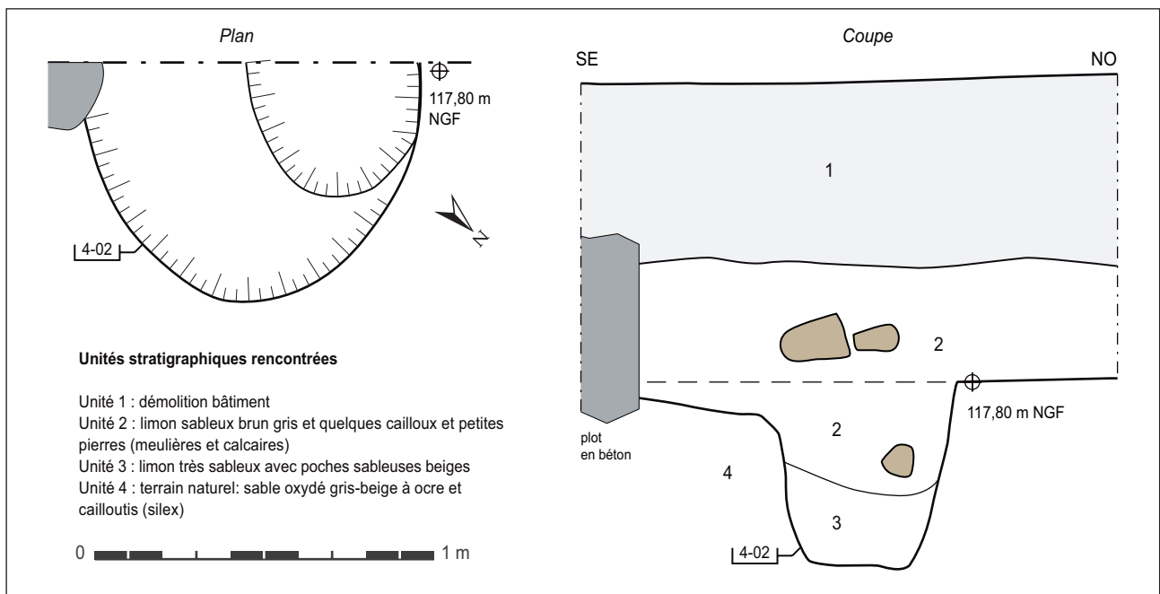
Fig. 44 Relevé en plan et coupe de la structure 4-02.
