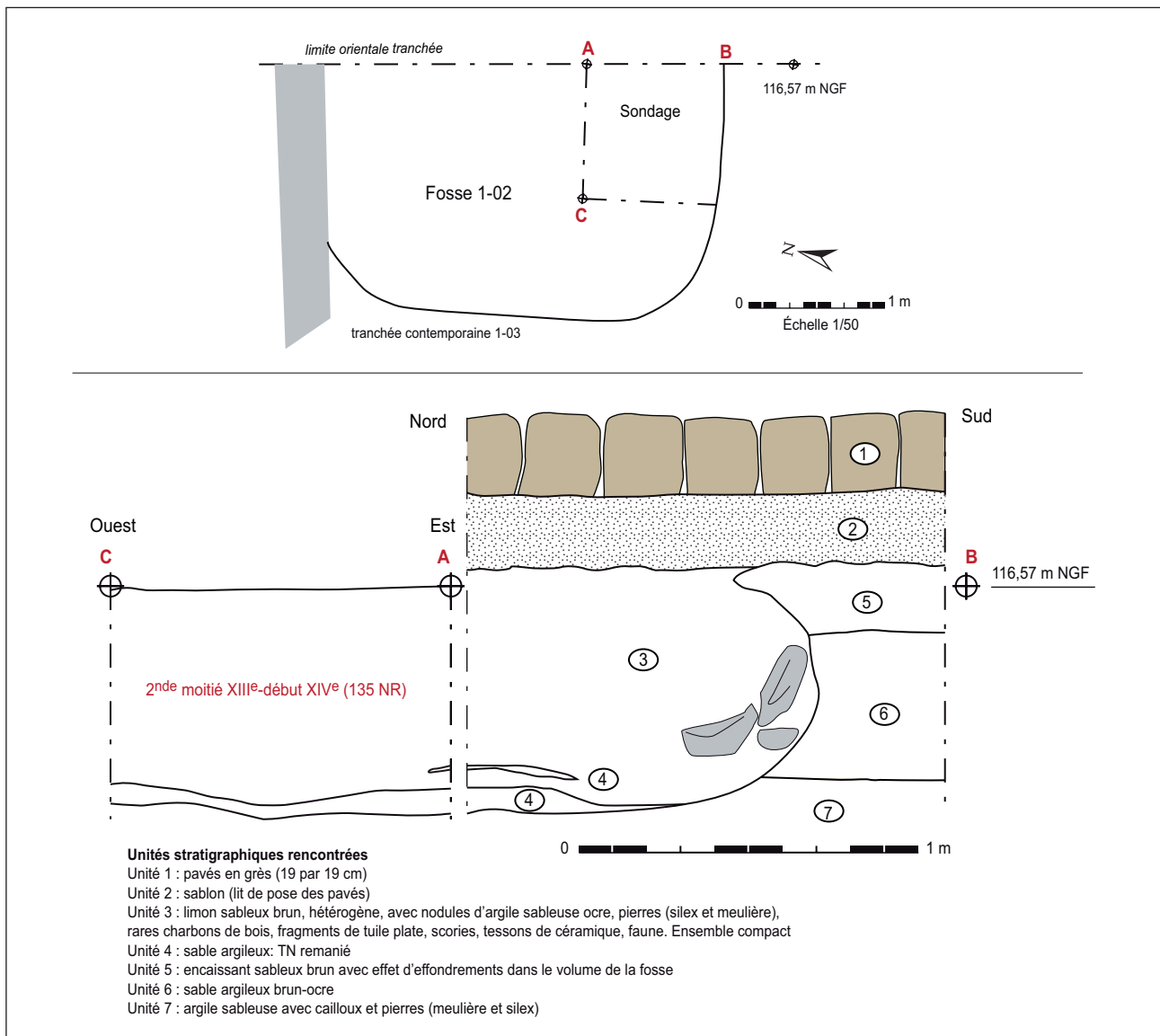
Fig. 22 Relevé en plan et coupe de la fosse 1-02. DAO N. Warmé, Inrap
