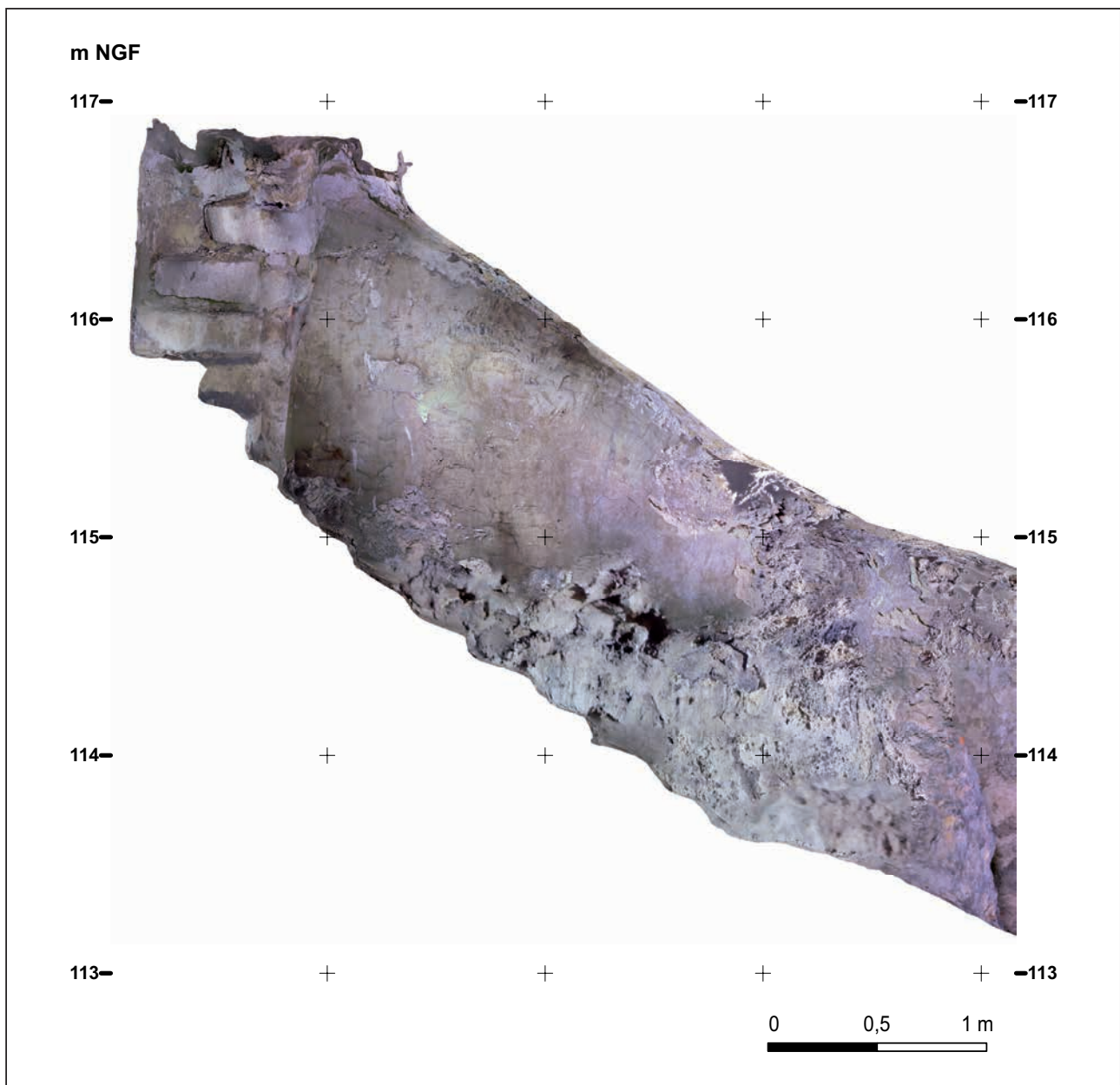
Fig. 88 Vue photogrammétrique de l'escalier.
