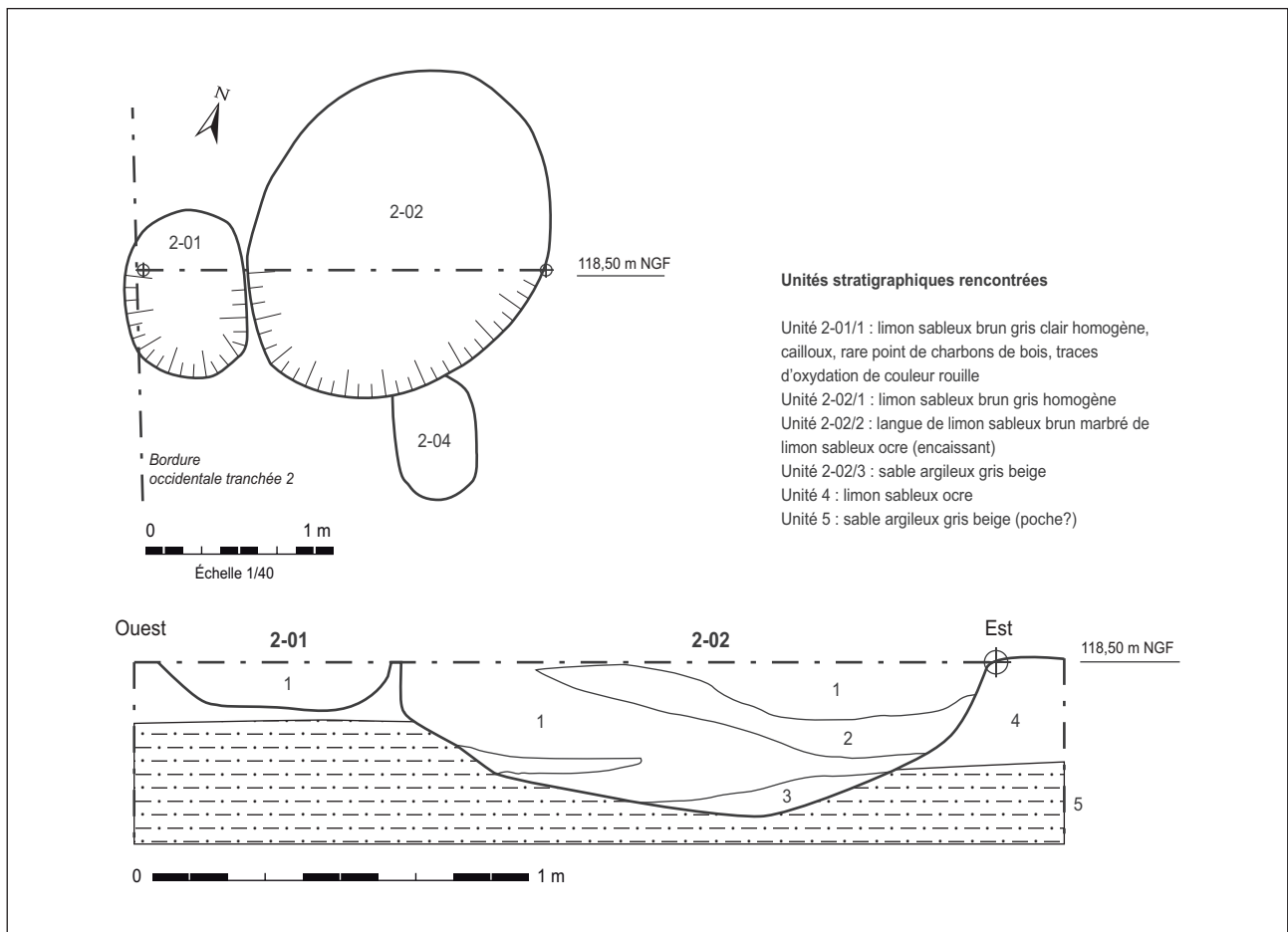
Fig. 25 Relevé en plan et coupe des fosses 2-01 et 2-02. DAO N. Warmé, Inrap
