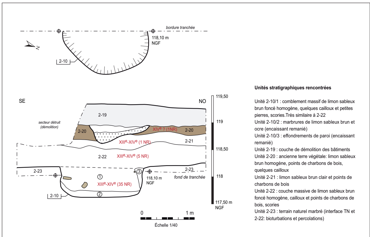
Fig. 27 Relevé en plan de la fosse 2-10 et relevé de la stratigraphie au droit de la fosse 2-10. DAO N. Warmé, Inrap
