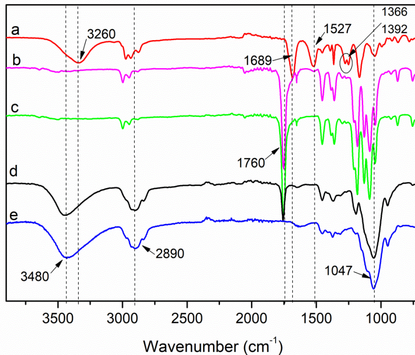
Fig. 4. FT-IR spectra of Boc-OH (a), Boc-NH-PLA (b), NH 2 -PLA (c), HPMC-PLA (d) and HPMC (e)
