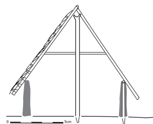
(b) hypothèse de restitution de l'élévation d'un bâtiment à murs porteurs en terre crue
