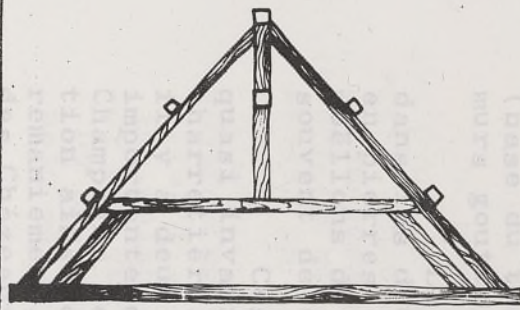
FERME b
