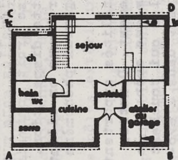
PLAN REZ DE CHAUSSEE
