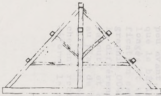
FERME a
