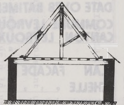
COUPE TRANSVERSALE EF
