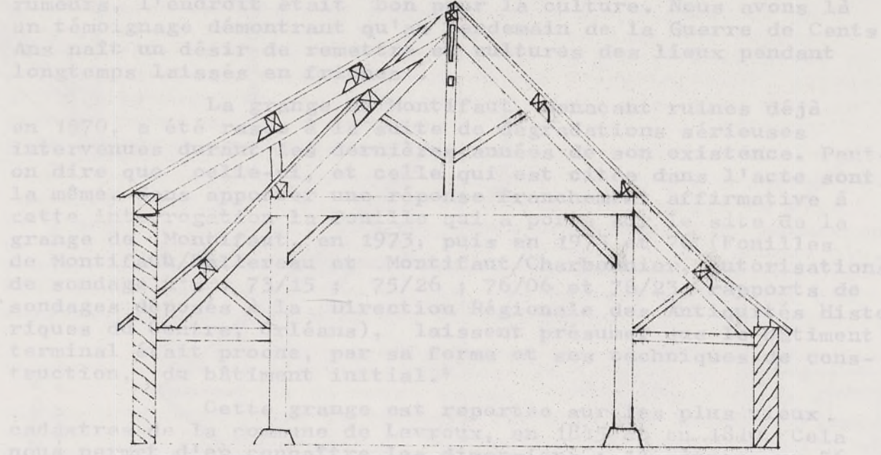
CHARPENTE DU COLOMBIER DE ROMSAC
