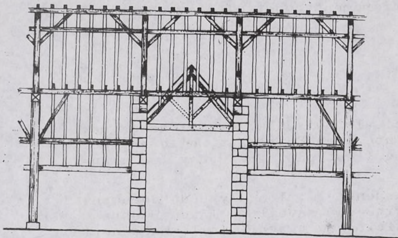
COUPE CC
