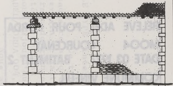
DETAIL FACADE NORD EST
