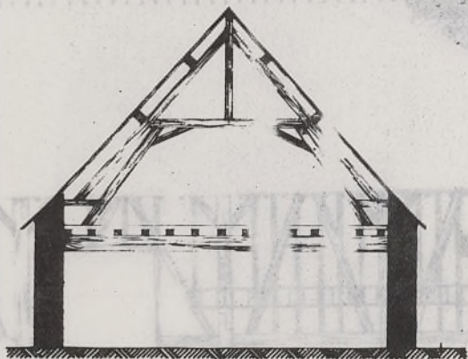
COUPE TRANSVERSALE AB
