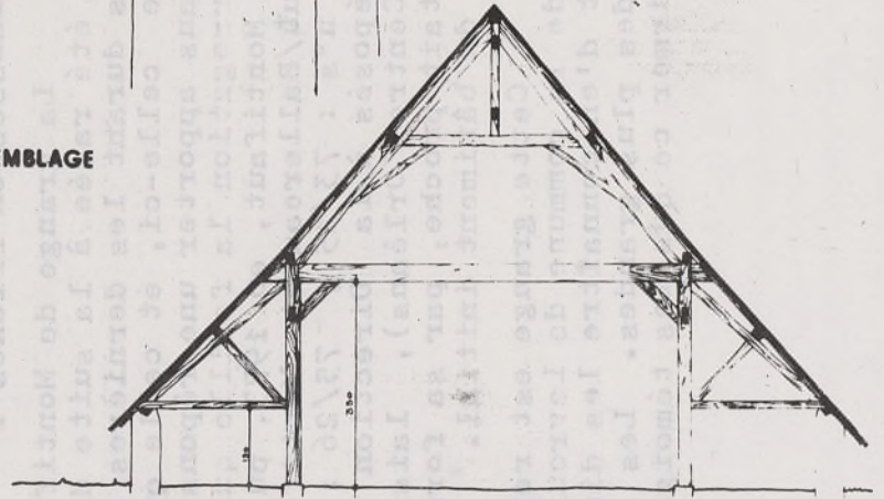
COUPE AA'
