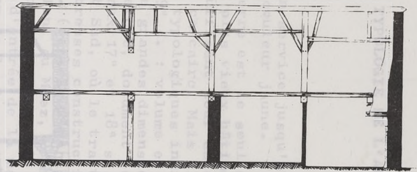
COUPE LONGITUDINALE AB
