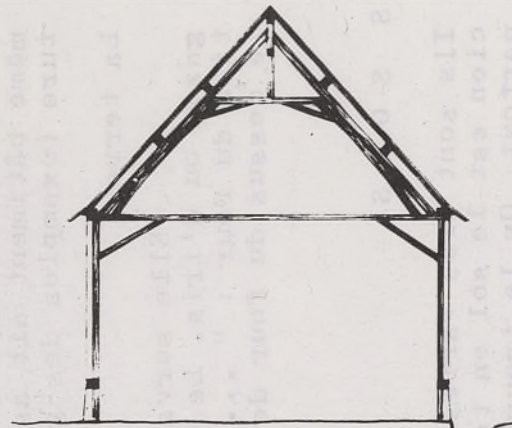
COUPE AB
