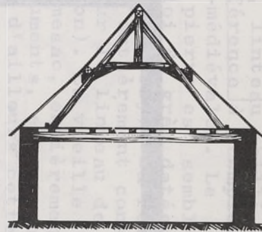
COUPE TRANSVERSALE CD
