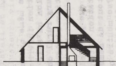
COUPE ab
