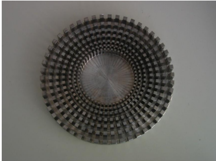
Figure 1 : Photographie de la cape d'invisibilité pour les vagues en vue de dessus ; Ce métamatériau de 20 centimètres de diamètre est constitué de 7 rangées concentriques de petits pylônes de 1 centimètre de haut. Quand les vagues pénètrent dans la cape, elles privilégient un trajet contournant la zone au centre du dispositif qui est donc protégée des vagues. (crédit photo : Photothèque CNRS, Institut Fresnel).
