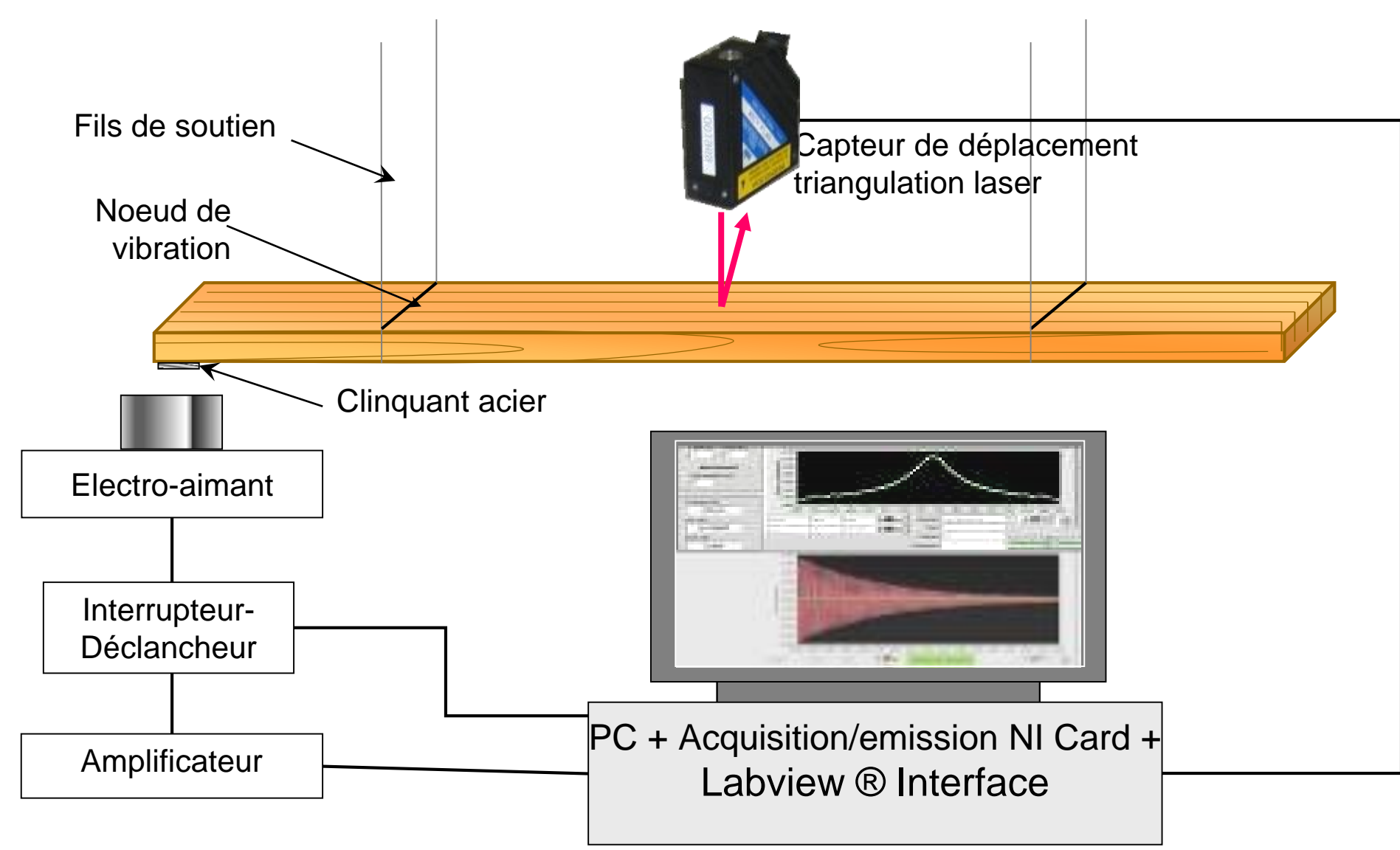
Schéma de principe du dispositif Vybris
