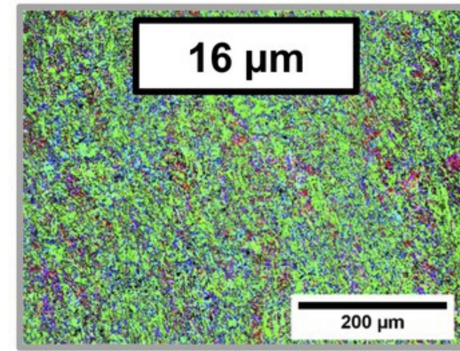
ECAP-RR (25 °C)
