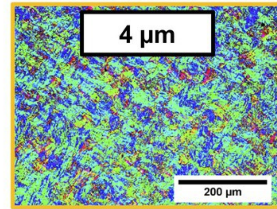
ECAP-RH (150 °C)
