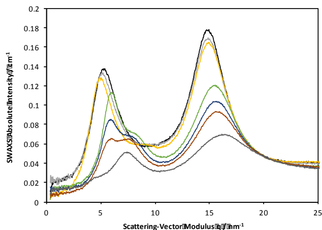
Figure 3. SWAXS patterns of [P_{4.4.4.4}][C_nCOO] -water mixtures, at: (—) x_w 0.00; (—) x_w 0.20; (—) x_w 0.41; (—) x_w 0.67; (—) x_w 0.75; (—) x_w 0.80; and (—) x_w 0.90.
