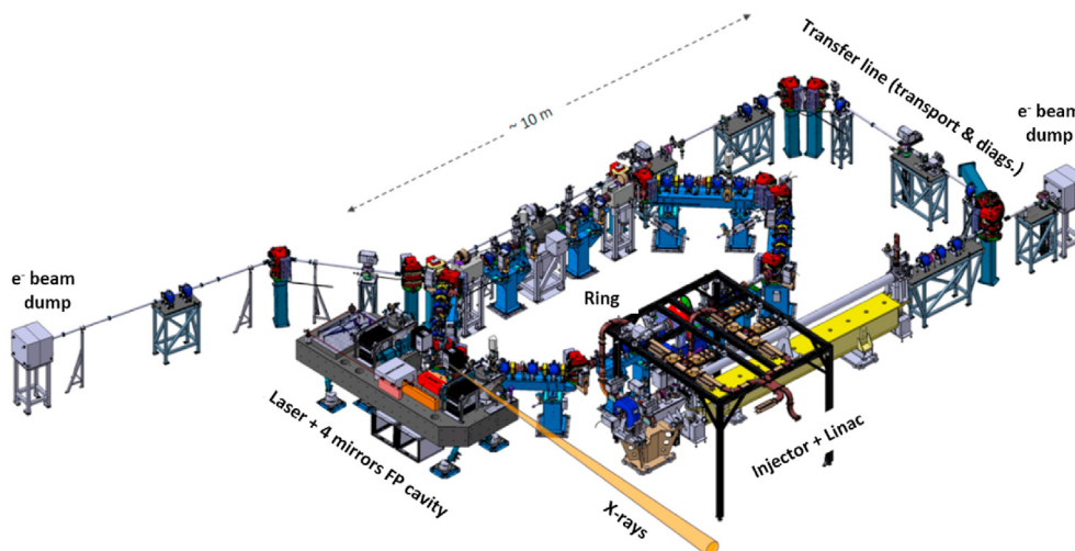
Fig. 1. ThomX layout.
