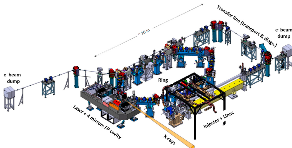
Fig. 1. ThomX layout.
