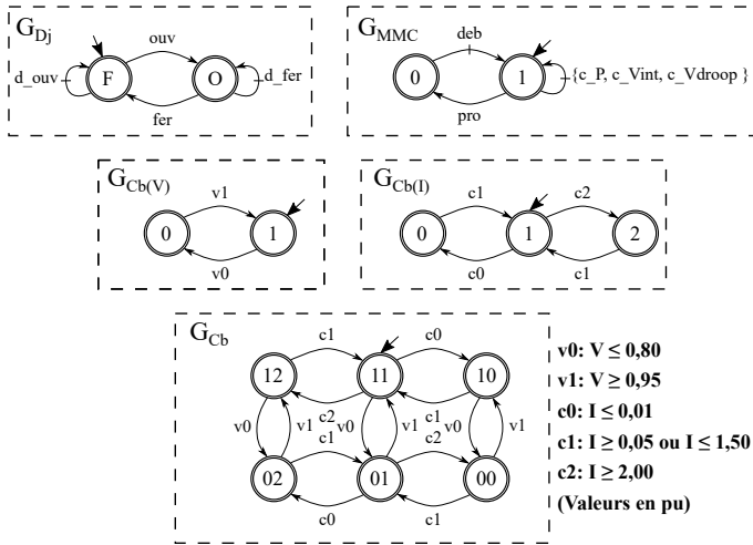
Fig. 6. Automates des composants du système : G_{Dj} , G_{Cb(v)} , G_{Cb(l)} , G_{Cb} .
