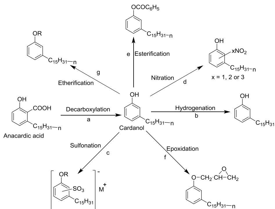
Figure 5 : Réactions sur le cardanol (a : décarboxylation ; b : hydrogénation ; c : sulfonation ; d : nitration ; e : estérification ; f : époxydation ; g : étherification)
