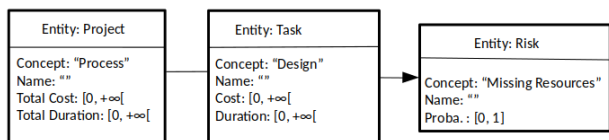
Figure 9 : Exemple de recherche de Connaissances Risque
