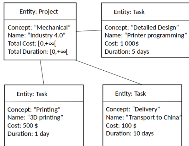
Figure 8 : Exemple de processus cible
