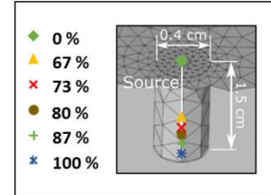
Figure 1 : Détail de l'électrode modélisée (modèle de la cellule conductrice).
