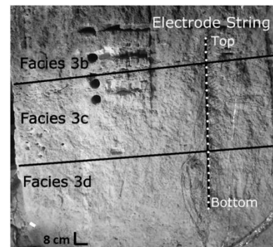
Figure 4 : Profil de micro-TRE à la paroi exposée aux feux. Les lignes noires délimitent les faciès 3b, 3c et 3d. Les points blancs repèrent électrodes.
