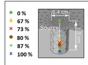
Figure 1 : Détail de l'électrode modélisée (modèle de la cellule conductrice).
