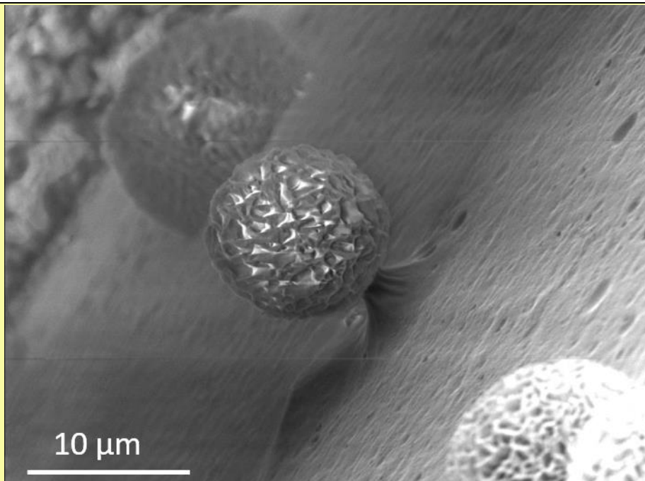
Figure 5: Observation en Microscopie électronique à balayage (MEB) de l'érosion de surface d'un film de PLA immergé dans une solution enzymatique. L'hétérogénéité de l'érosion conduit, dans ce cas, au relargage de sphérulites de taille typique la dizaine de microns [17].
