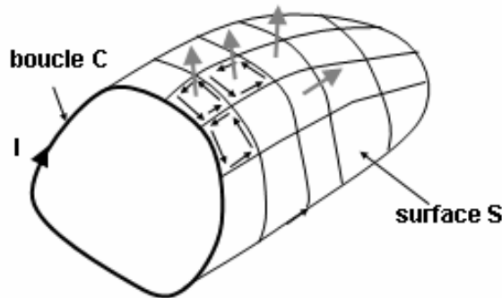
Figure 2. Equivalence entre un courant circulant dans une boucle et une densité surfacique de dipôles normaux
