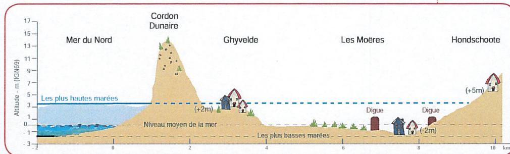
Figure 5.47 : Localisation des waterings de la plaine maritime flamande et coupe transversale du polder au nord-est de Dunkerque (AGUR, 2014 d'après IIW)
