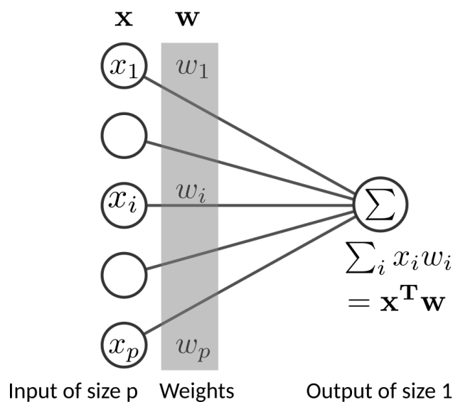
Fig. 3: Linear regression
