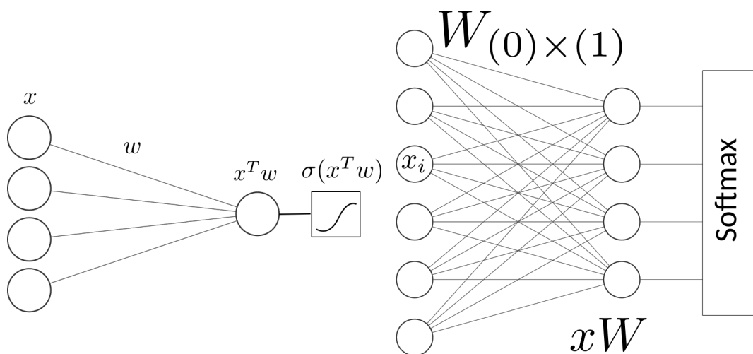
Input layer of size (0) Output layer of size (1) Input layer of size (0) Output layer of size (1)
