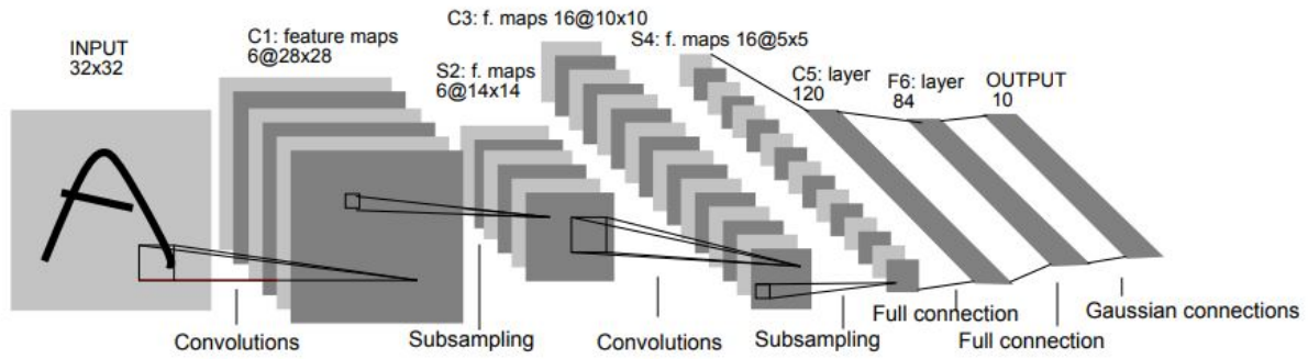
Fig. 2: LeNet
