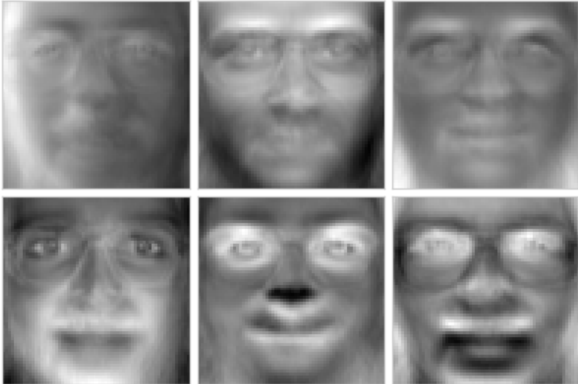
PCA first 6 loadings
