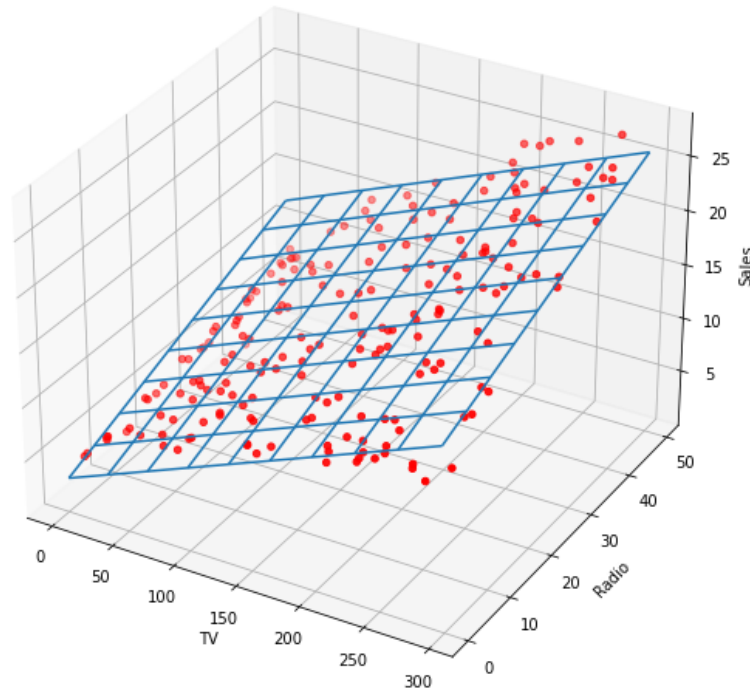
Fig. 4: Linear regression
